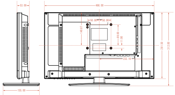
《寸法図》
